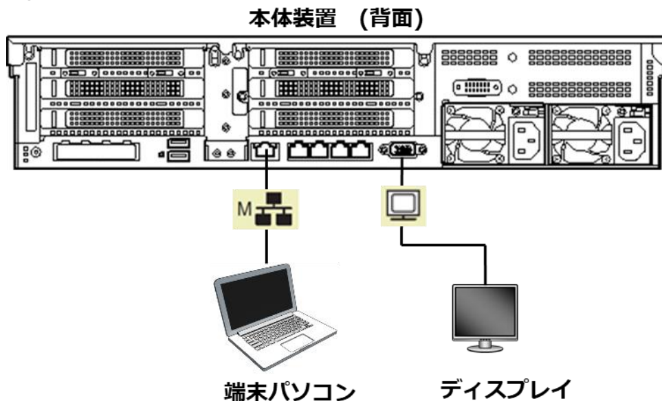
5 Figure 4-1 接続図
