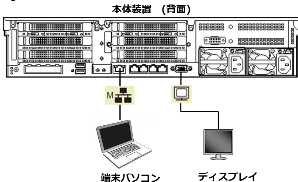
15 Figure 4-1 接続図
