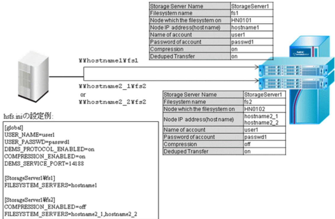
図 5-1 ユニバーサル高速 I/O モジュール設定ファイルの設定例
