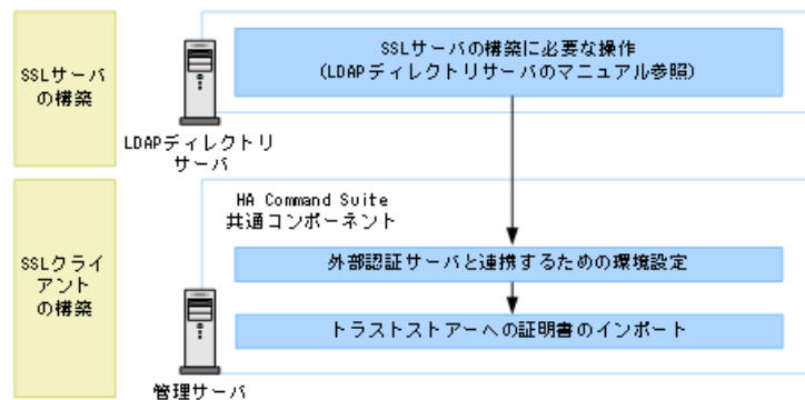
図 5-4 LDAP ディレクトリサーバと管理サーバ間のセキュリティ通信のための操作フロー
