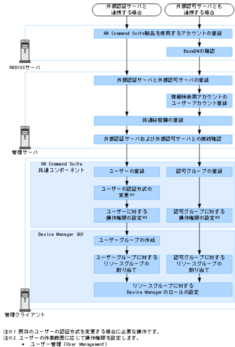
図4-2 RADIUSサーバでユーザー認証するための操作フロー
