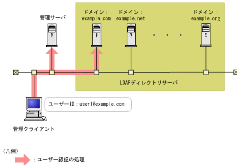
図 4-6 マルチドメイン構成のユーザー認証処理（ドメイン名を含んでいるユーザー ID の場合）
