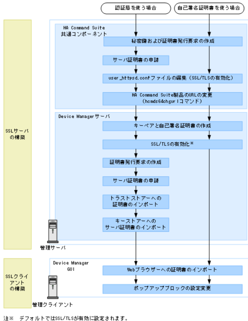
図 5-3 管理サーバと管理クライアント（GUI）間のセキュリティ通信のための操作フロー
