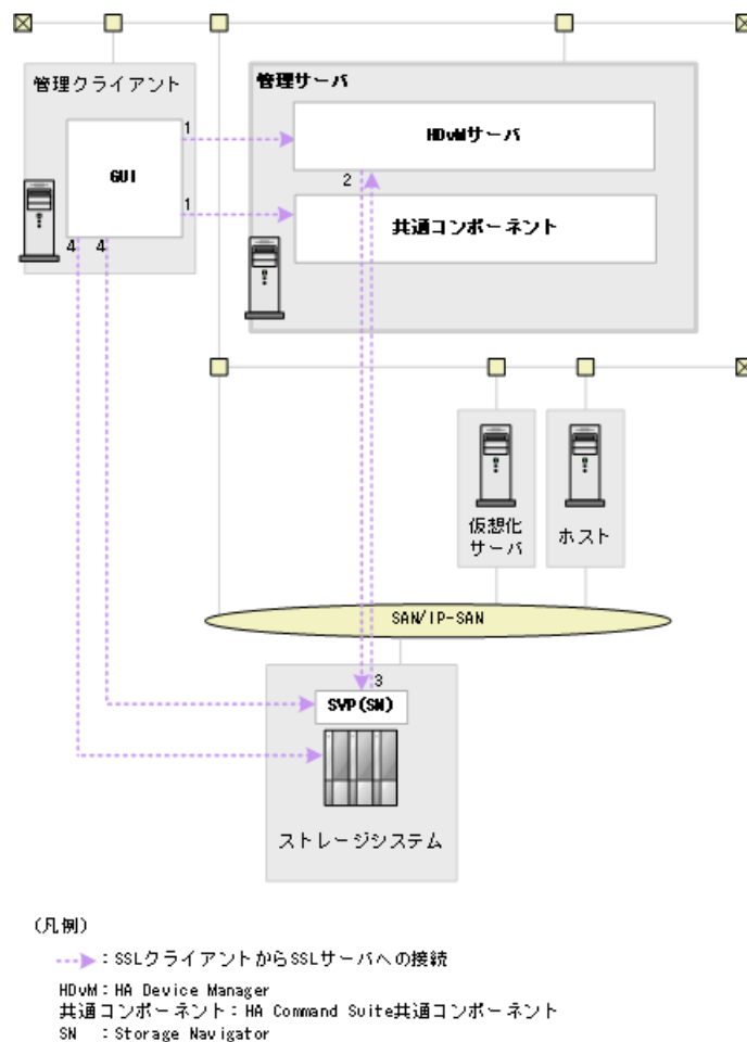
図 5-1 Device Manager のセキュリティ通信路 (1/2)
