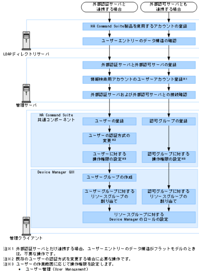
図 4-1 LDAP ディレクトリサーバでユーザー認証するための操作フロー
