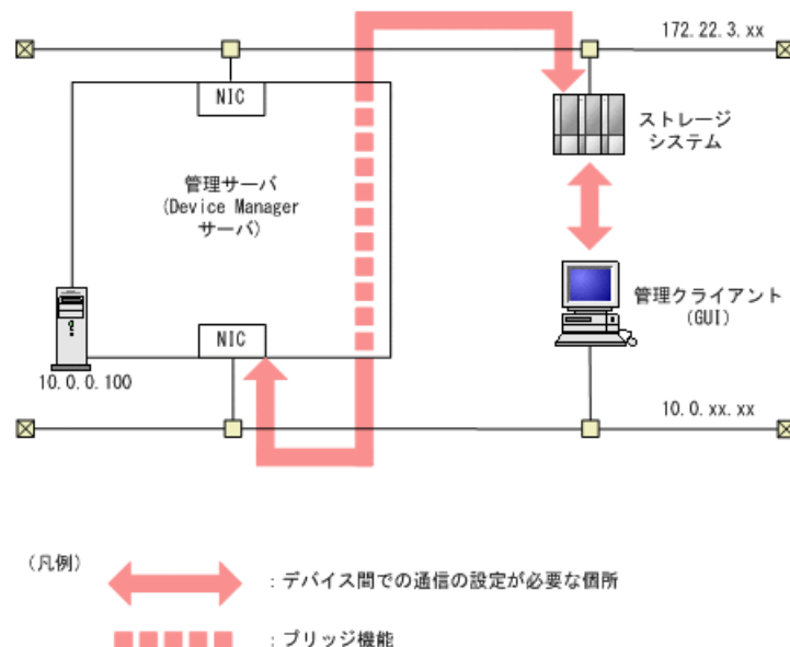
図 2-1 管理サーバのブリッジ機能を使用したネットワークの構成例
