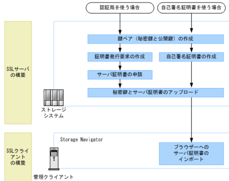
図 5-6 ストレージシステムと管理クライアント（GUI）間のセキュリティ通信のための操作フロー
