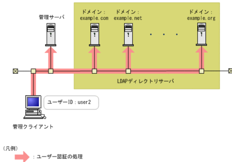
図 4-7 マルチドメイン構成のユーザー認証処理（ドメイン名を含んでいないユーザー ID の場合）
