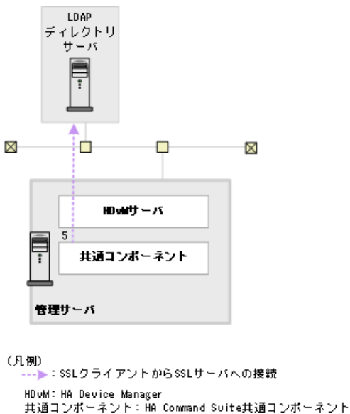
図 5-2 Device Manager のセキュリティ通信路 (2/2)
