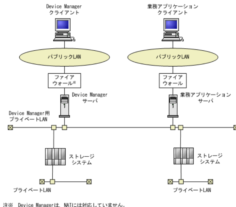
図 1-2 管理用の LAN を分離し、ファイアウォールを設置した構成
