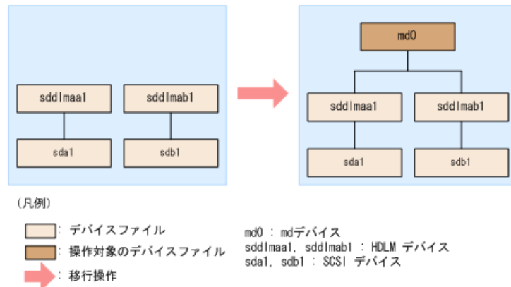
図3.10 HDLMデバイス上にmdデバイスを作成した場合のデバイス構成
