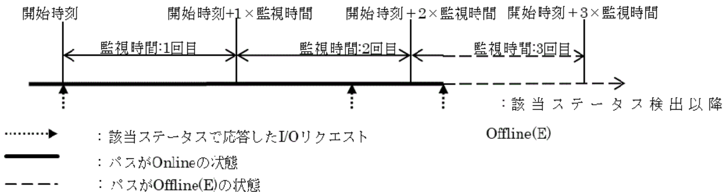
図2.18 リトライ回数監視機能でパスを閉塞しない場合
