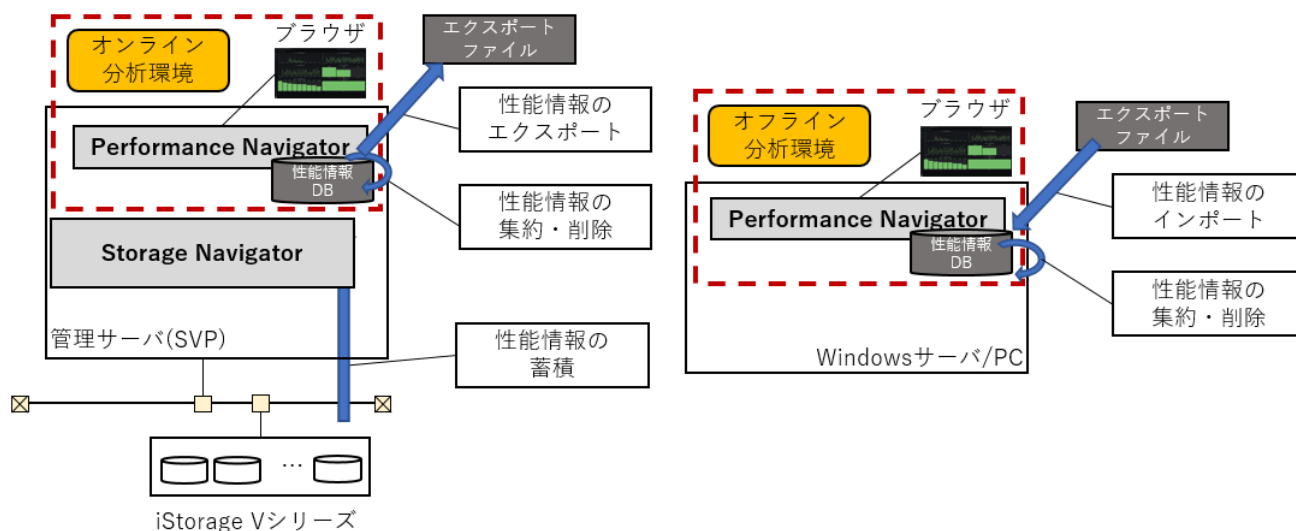
図 4-1 性能情報の管理
