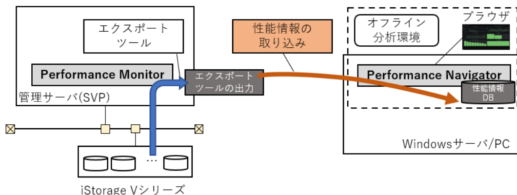
図 3-30 Performance Monitor との併用運用
