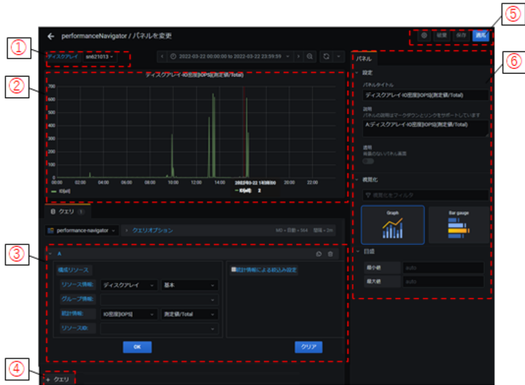
図 B-6 パネル変更画面
