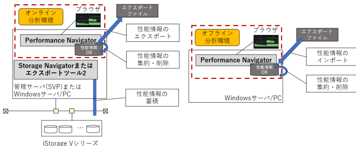
図 4-1 性能情報の管理
