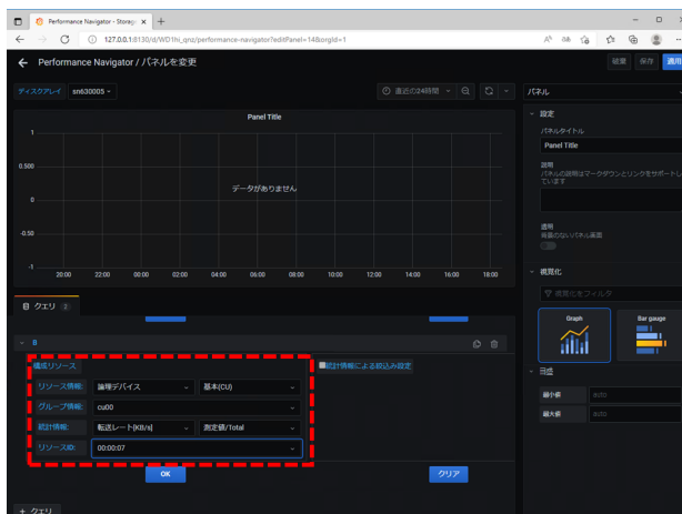
図 4-13 任意のリソースの選択(3)
