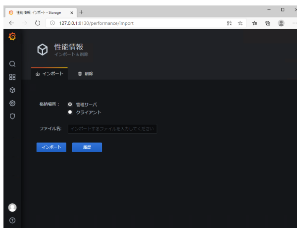
図 3-15 「性能情報」のインポート
