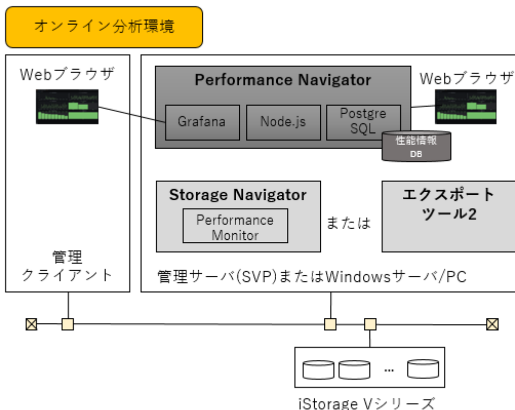
図 1-4 オンライン分析環境のシステム構成
