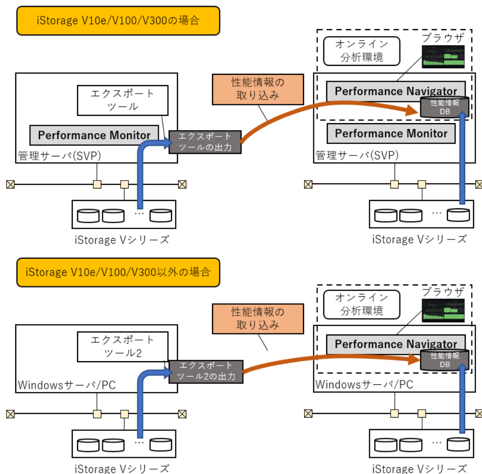
図 3-29 Performance Monitor またはエクスポートツール 2 からの移行運用
