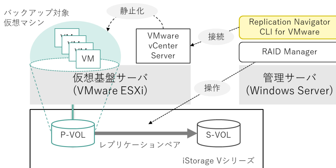
図 1.1.1 Replication Navigator CLI for VMware の動作イメージ
