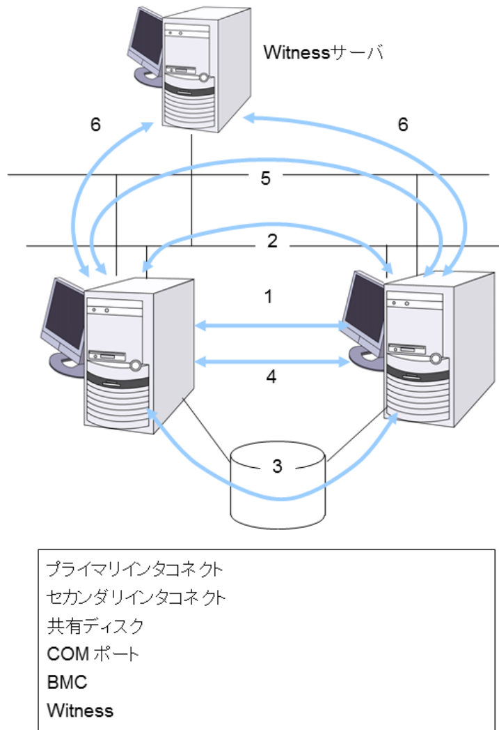
図 3.2 サーバ監視
