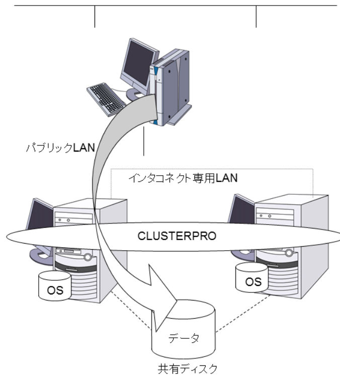
図 3.4 システム構成
