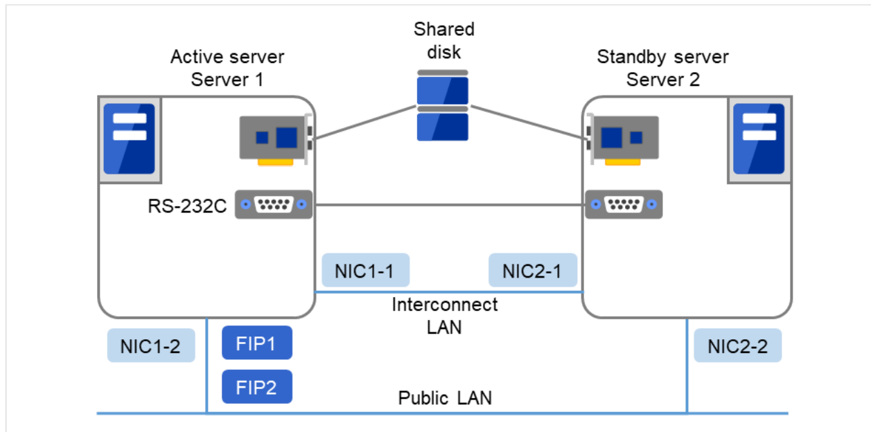
図 3.18 クラスタ構成例（共有ディスク型）
