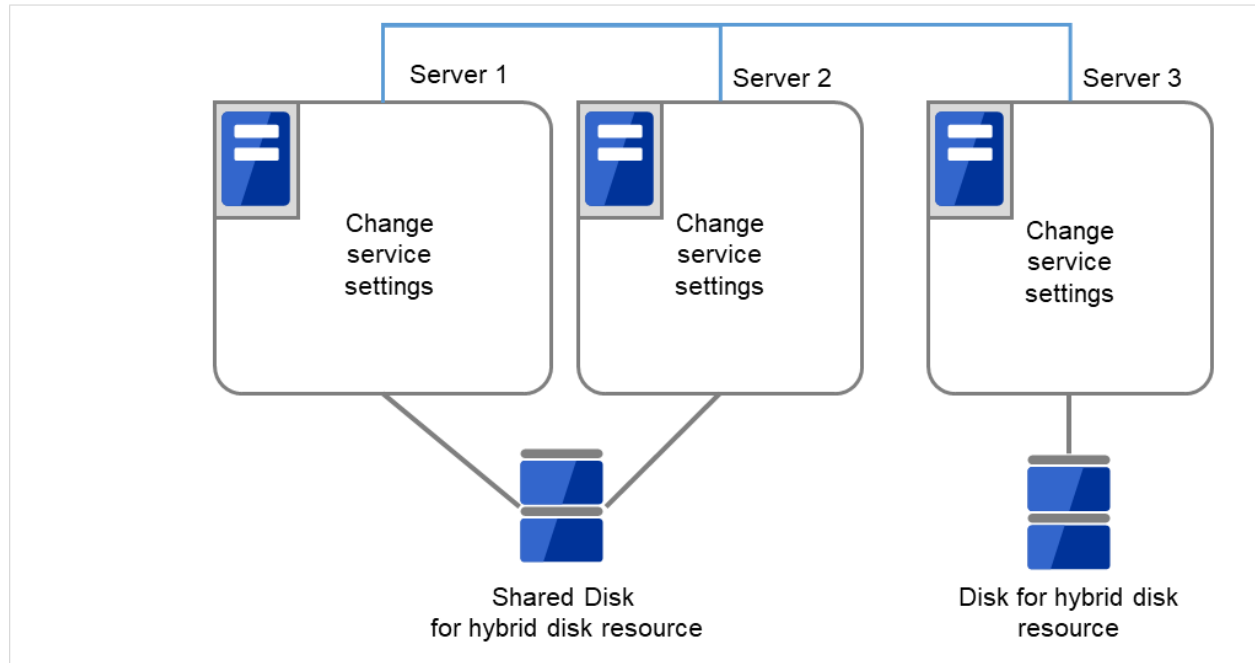
図 2.70 CLUSTERPRO サービスが起動しないよう設定変更
