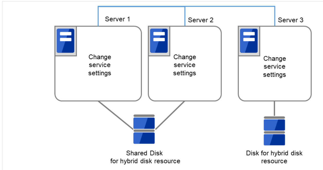
図 2.58 CLUSTERPRO サービスが起動しないよう設定変更
