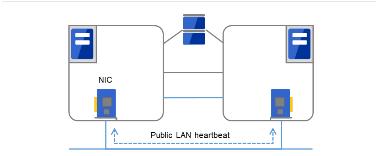
図 3.3 LAN ハートビート/カーネルモード LAN ハートビート (セカンダリインタコネク)
