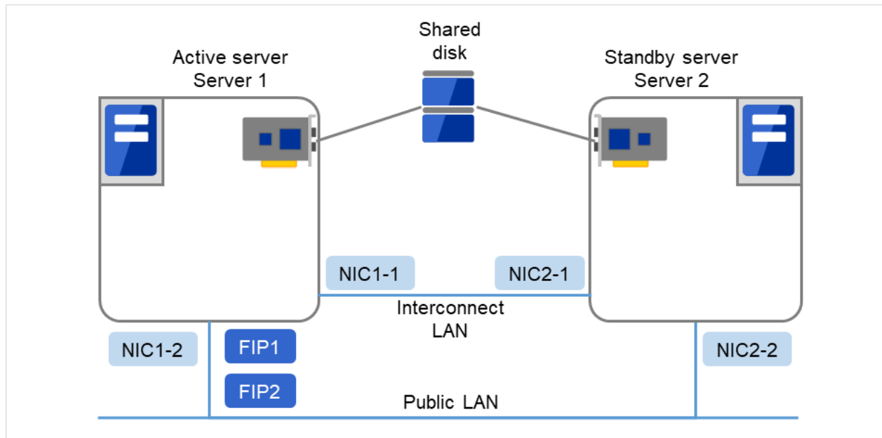
図 6.5 2 ノードクラスターの例 (ボリュームマネージャリソース使用時)
