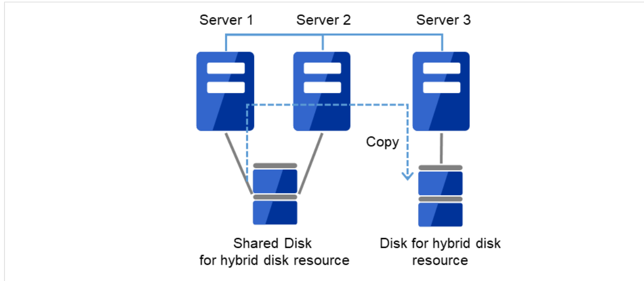
図 2.23 Server1 よりミラー復帰開始 (差分コピー)
