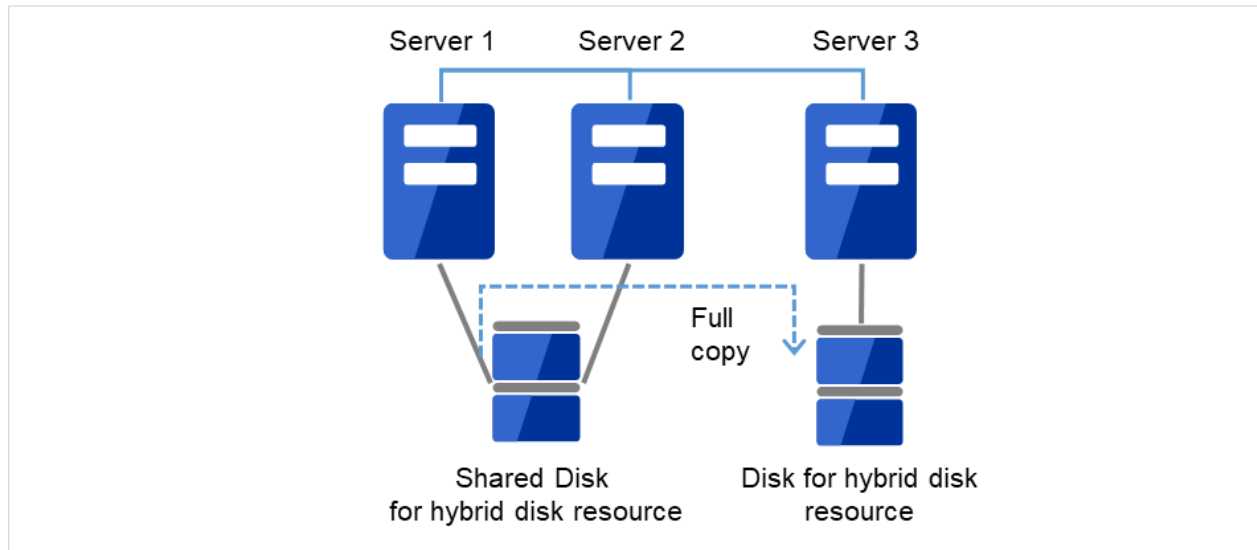
図 2.13 Server1 よりミラー復帰開始（全面コピー）
