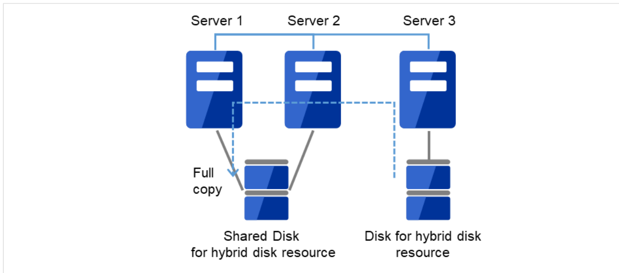
図 2.20 ミラー復帰開始（全面コピー）
