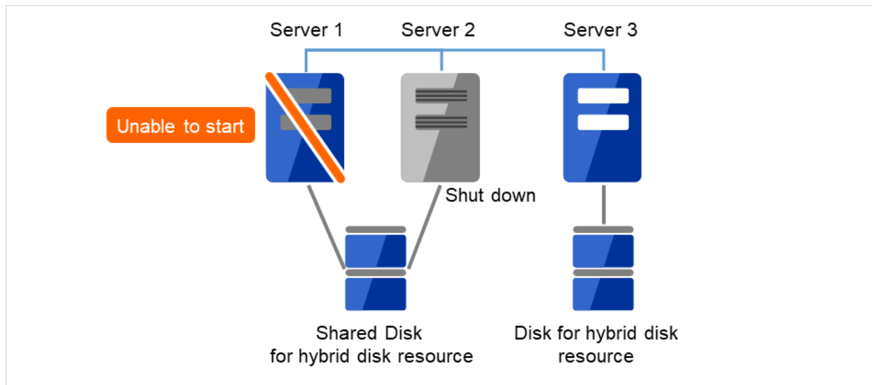
図 2.15 Server2 をシャットダウン
