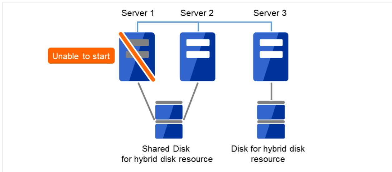
図 2.14 Server1 が起動できず、共有ディスクも使用できない
