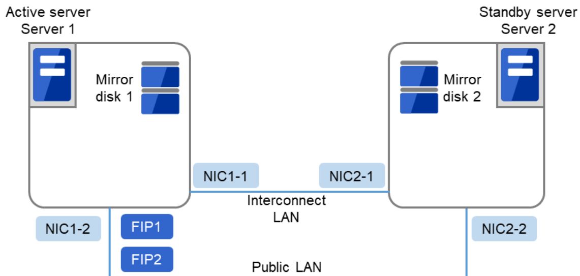
図 3.17 クラスタ構成例 (1) (ミラーディスク型)
