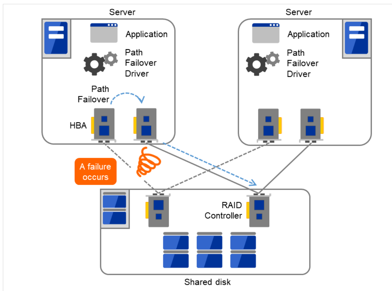
図 2.13 パスフェイルオーバードライバ
