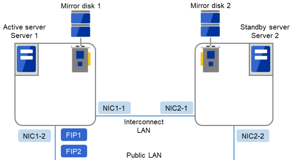
図 3.19 クラスタ構成例 (2) (ミラーディスク型)
