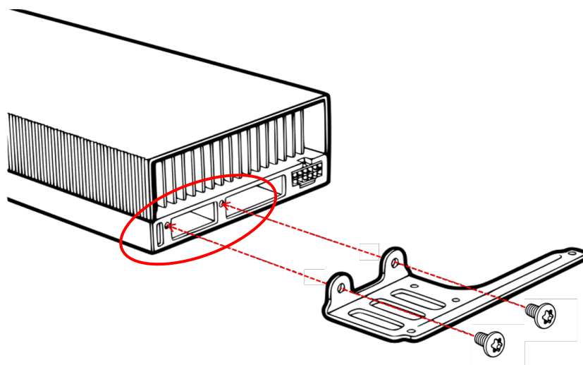
ボード後部 リテーナー(GPU エクステンダ)取り付け前
