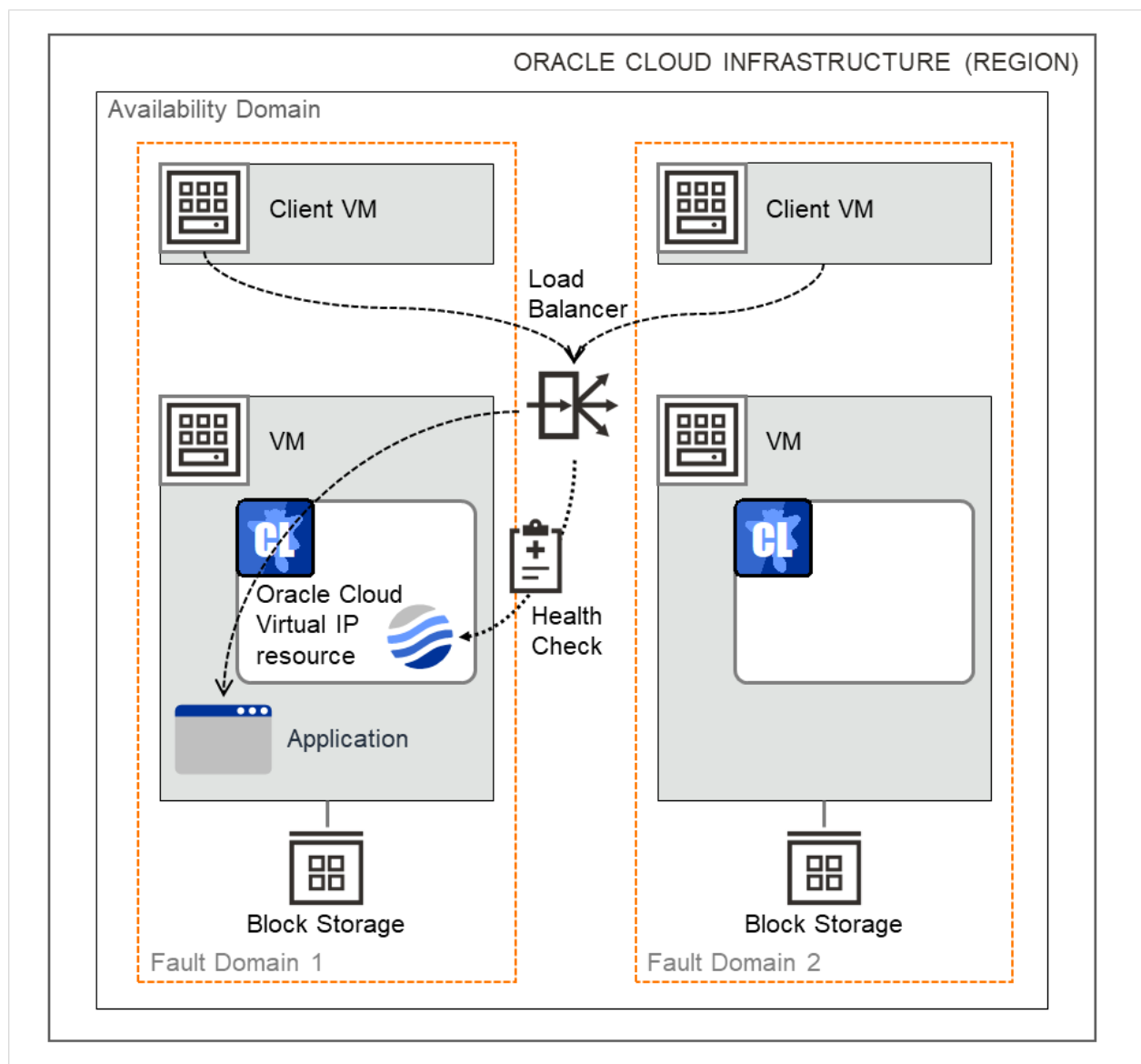
図 3.119 Oracle Cloud 仮想 IP リソースを使用する構成（プライベートロードバランサ）
