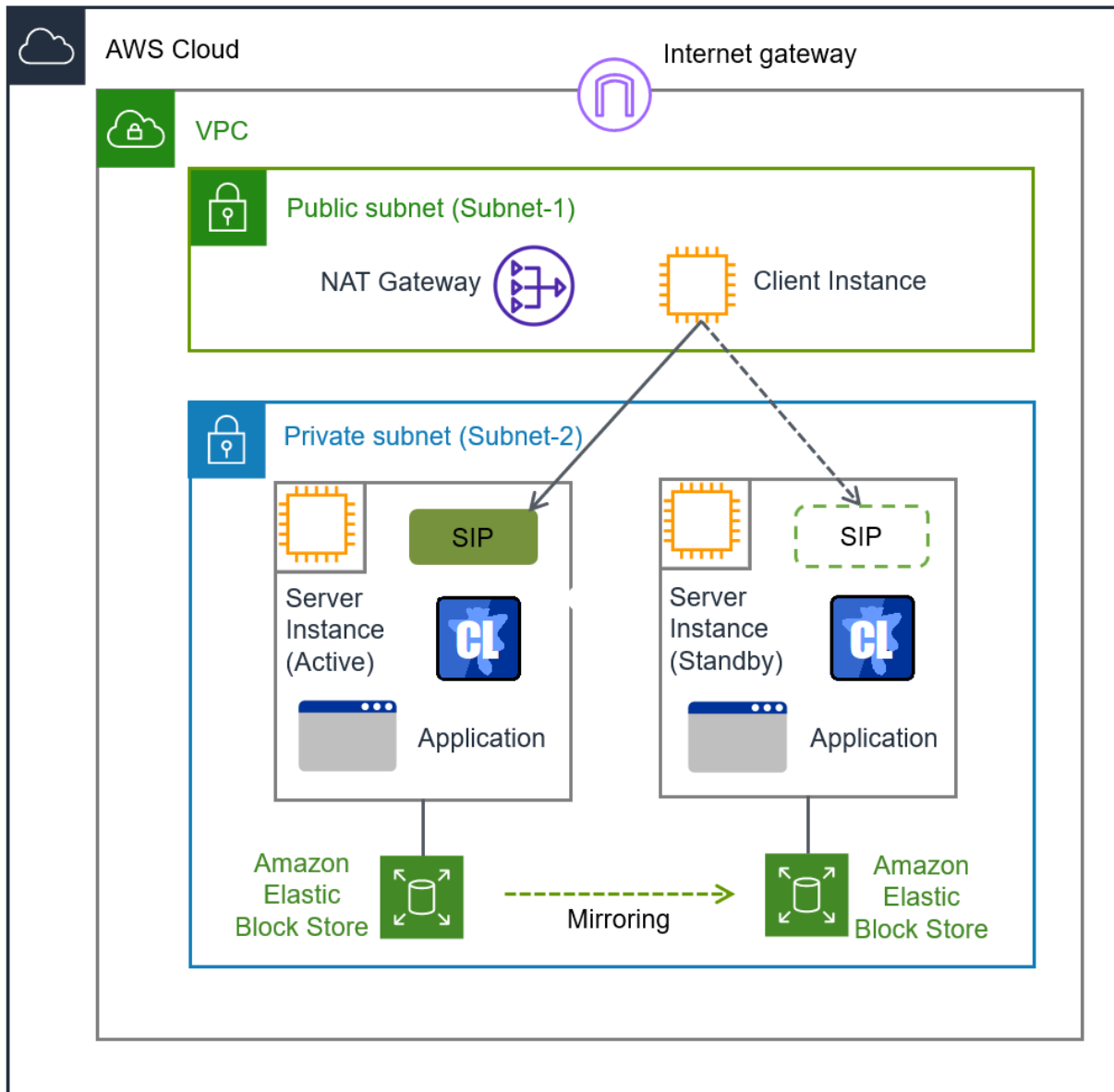
図 3.112 AWS セカンダリ IP リソースを使用する構成
