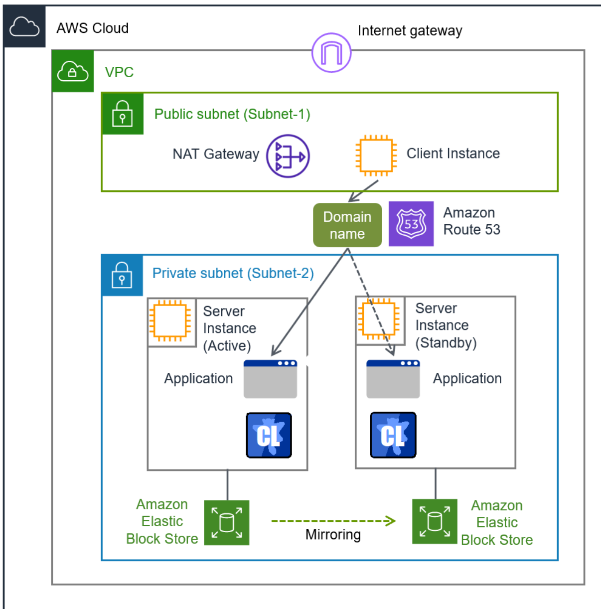
図 3.113 AWS DNS リソースを使用する構成
