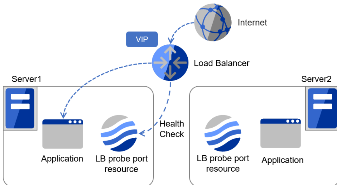
図 3.109 LB プローブポートリソースを使用する構成
