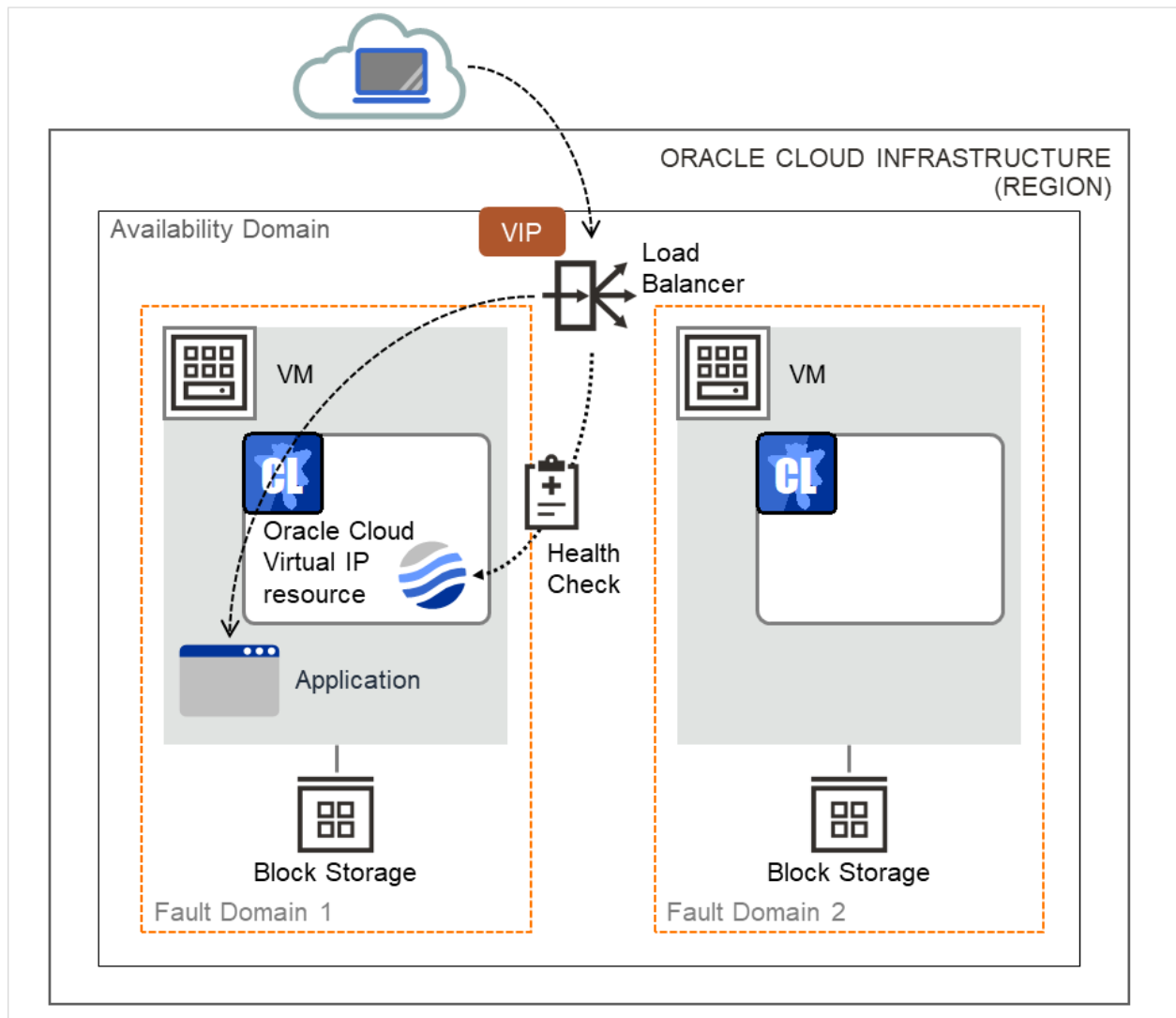
図 3.118 Oracle Cloud 仮想 IP リソースを使用する構成
