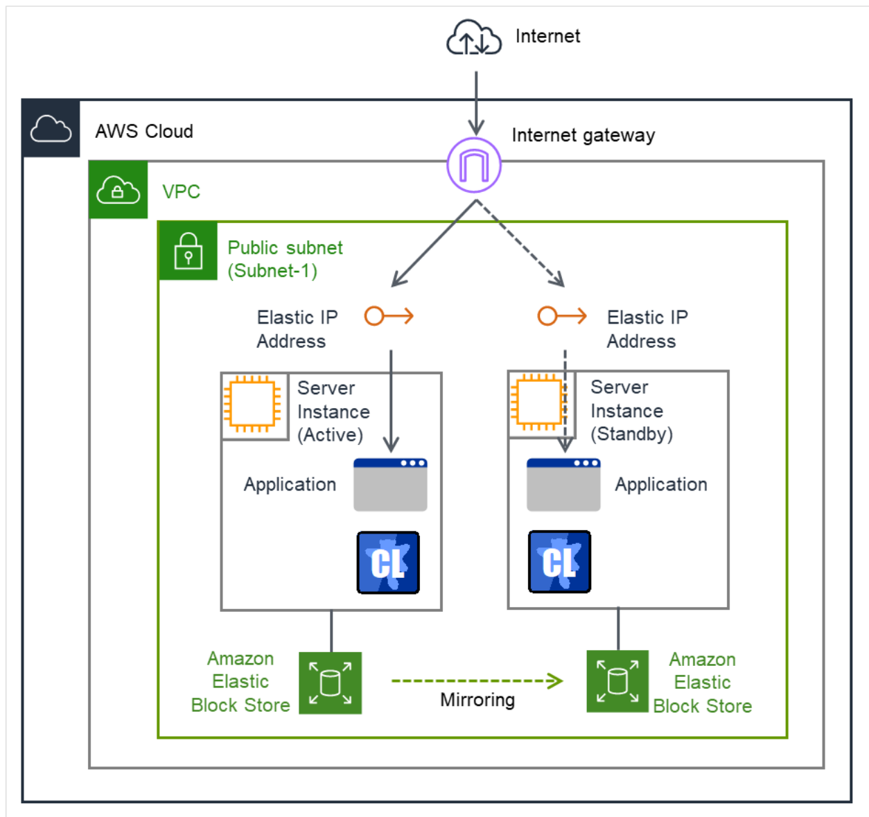
図 3.110 AWS Elastic IP リソースを使用する構成
