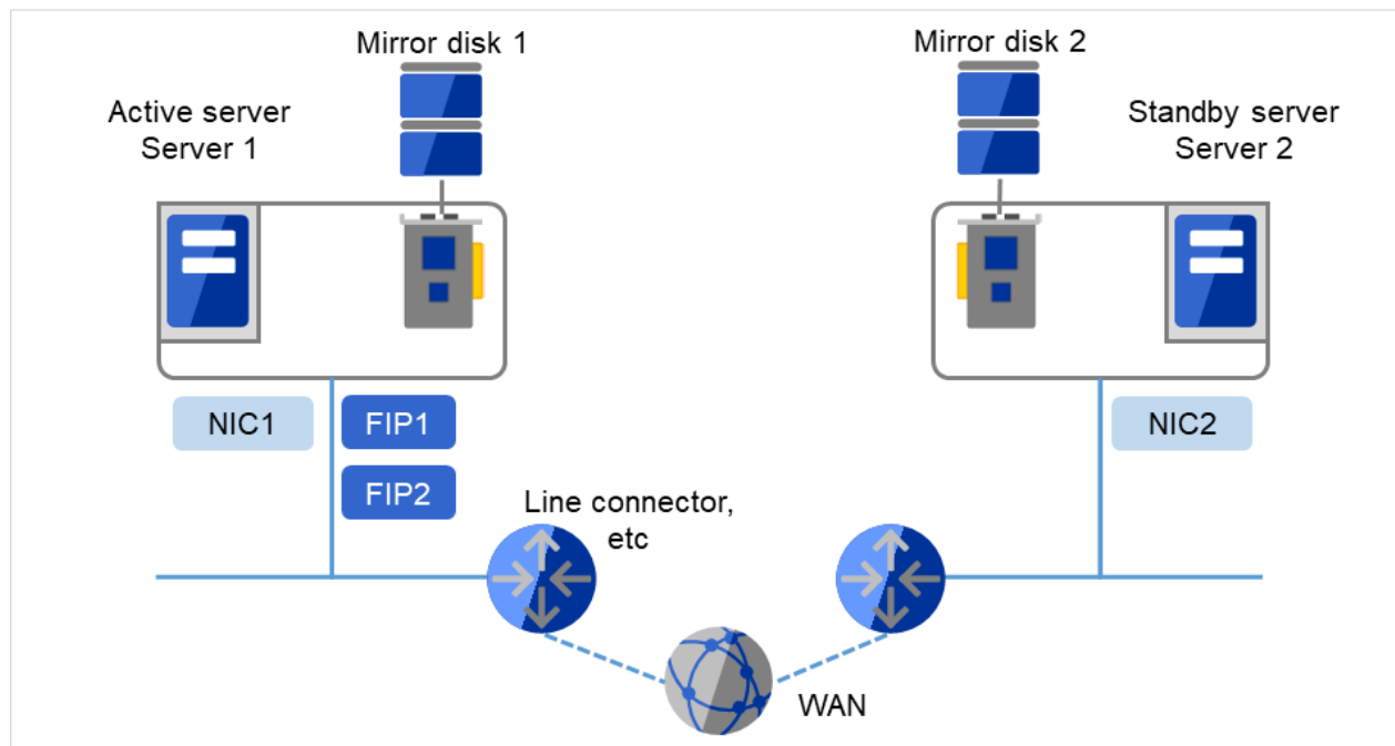
図 6.4 2 ノードクラスターの例（遠隔構成ミラーディスクリソース使用時）
