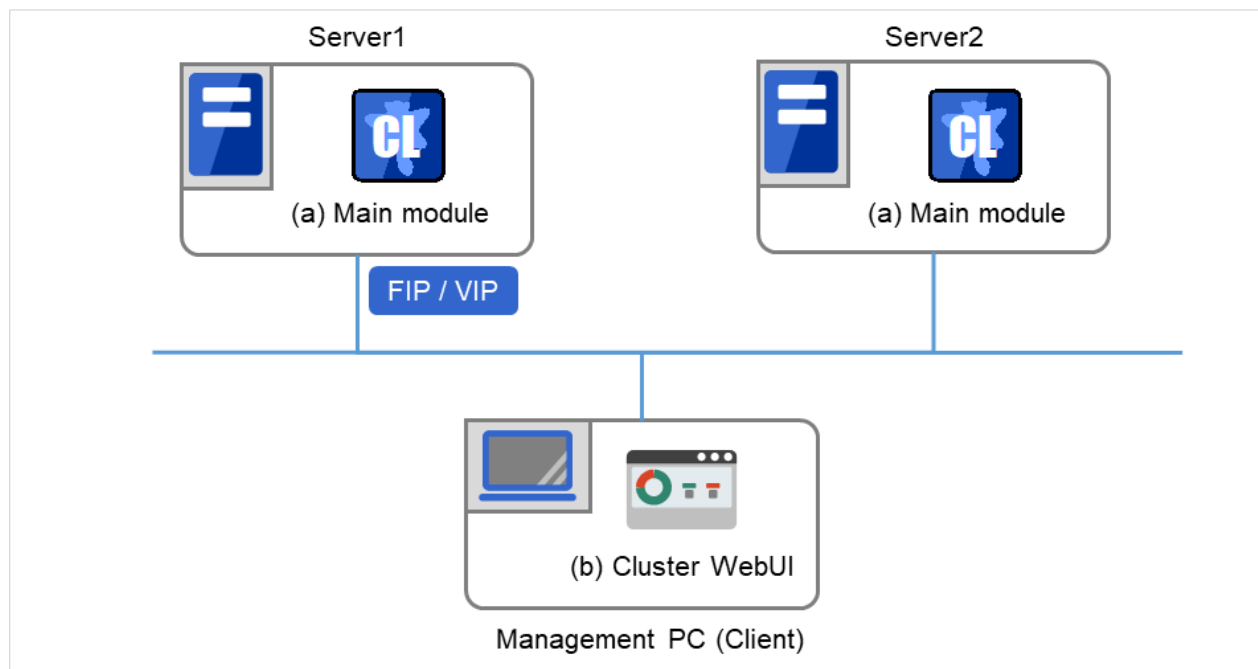
図 6.1 Cluster WebUI
