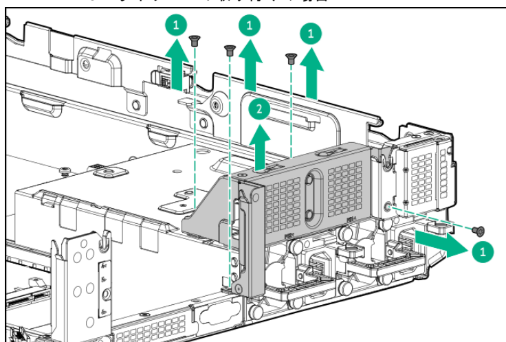
3rd ライザーへの取り付けの場合
