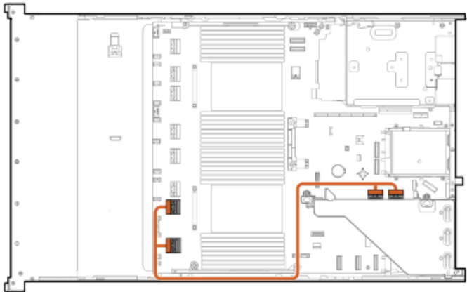
ケーブル配線図
