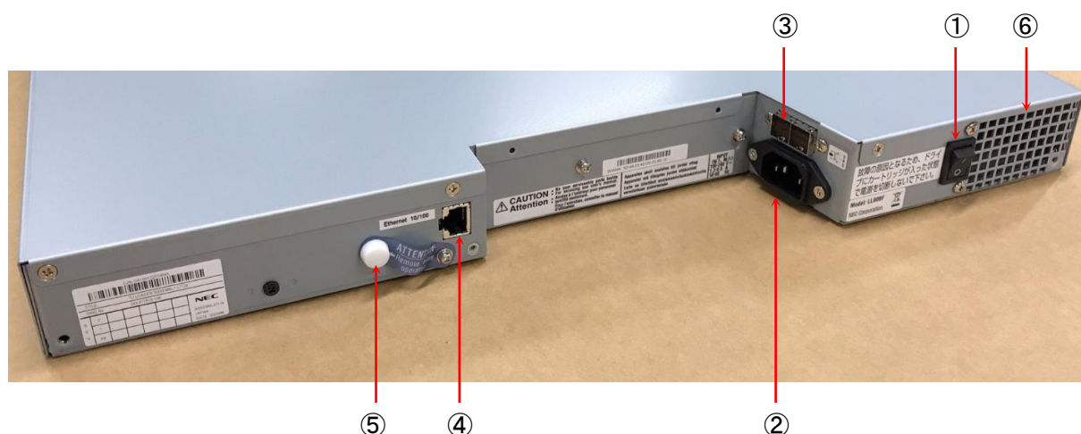
図 1-2 装置背面
