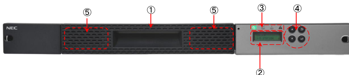
図 1-1 装置前面
