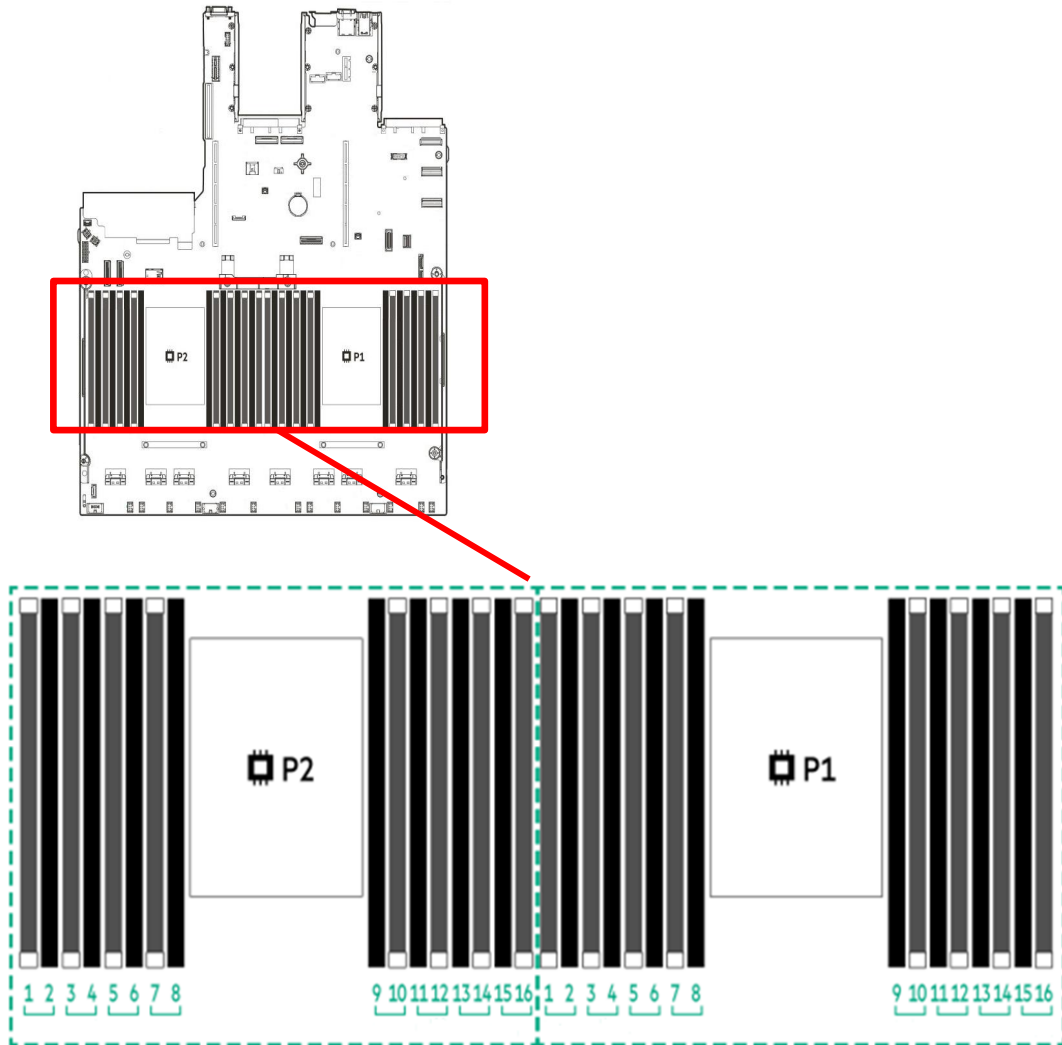
装置前面側
