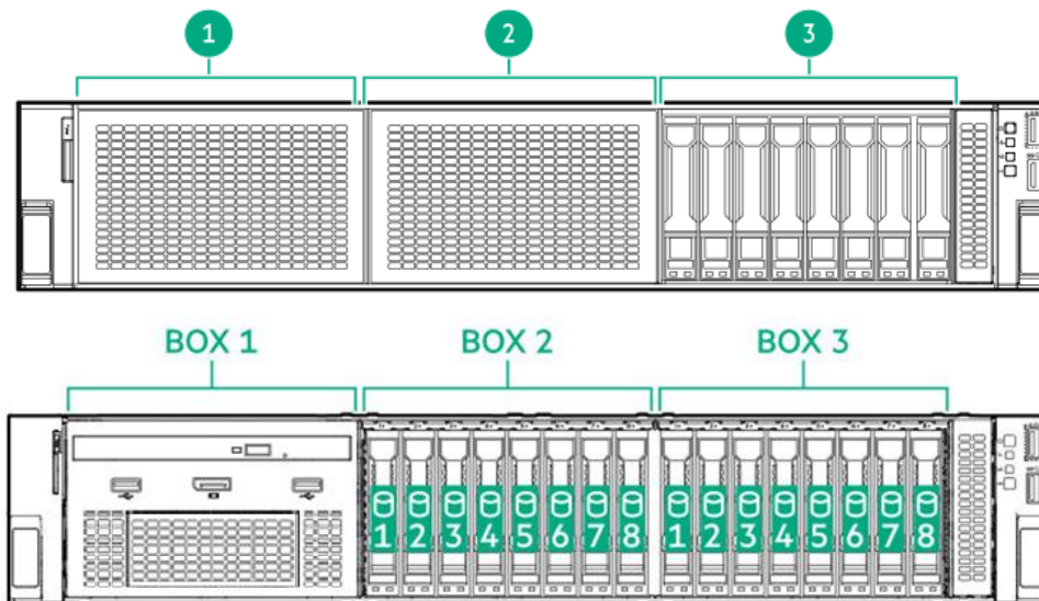
8x 2.5 型ドライブモデル フロント BOX
