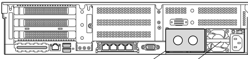
増設スロット 標準スロット
